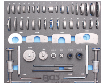
BGS1102 50 ST. / PCS. Terugstelset remzadelzuigers links-rechts 50-dlg. Set d'outils repousse piston de freins gauche-droite 50pcs 193 €
