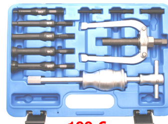
BGS7710 Trekkerset voor binnen lagers Jeu d'extracteurs de roulements intérieurs Ø 8-34mm
