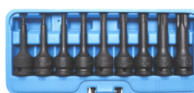
Versterkte doppen Douilles impact 1/2 L=75mm BGS5480 T20 - T70 61 € BGS5481 IN5 - IN19 61 € BGS5482 XZN M6 - M16 62 € BGS5483 RIBE M5-M14 62 €
